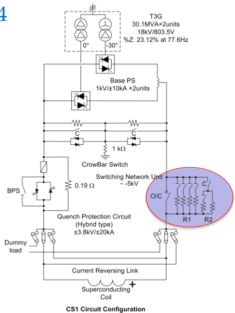
CS1 Circuit Configuration Alimentazione di CS con SNU
