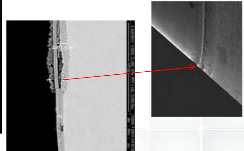
5000 ore di esposizione al piombo liquido @500° C nell'impianto CHEOPEIII
