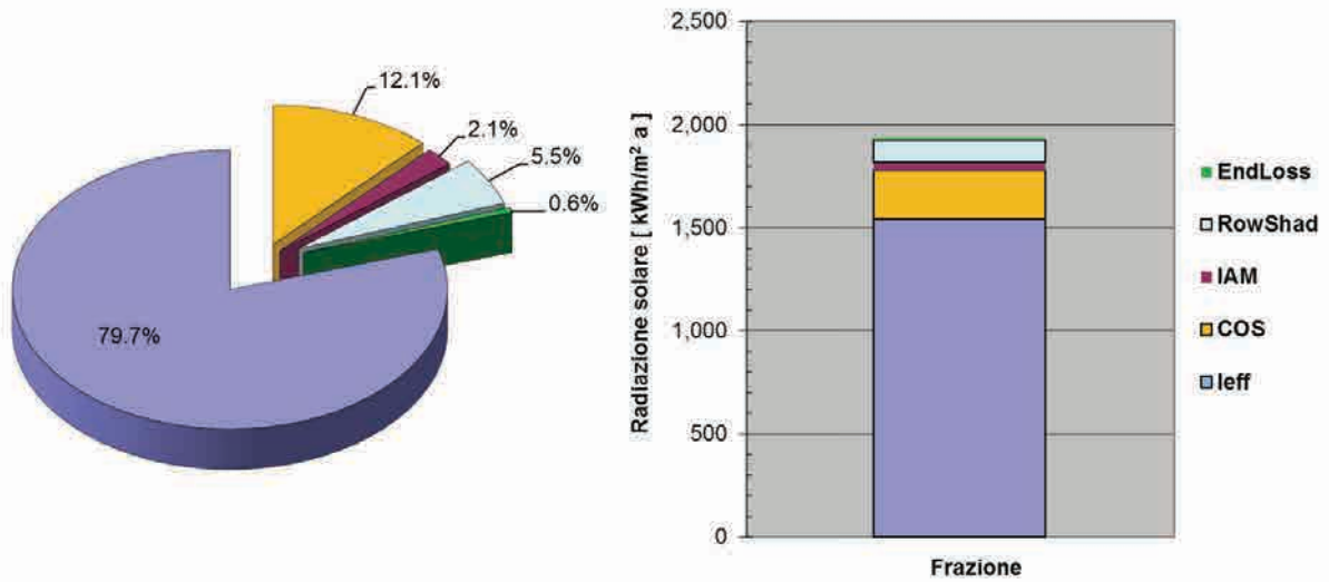
Figura 13: Distribuzione delle differenti componenti della radiazione solare
