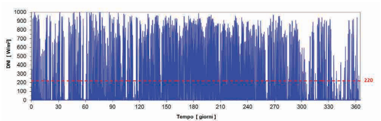
Figura 4: Distribuzione oraria della radiazione solare diretta (DNI)
