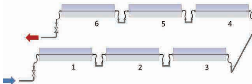
Figura 19: Schematizzazione stringa di collettori solari
