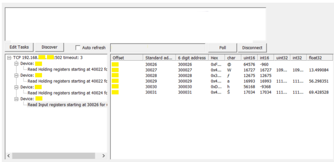
Figura 34. Misure di temperatura ambiente e RH su Address 30026/7 e 30030/1
