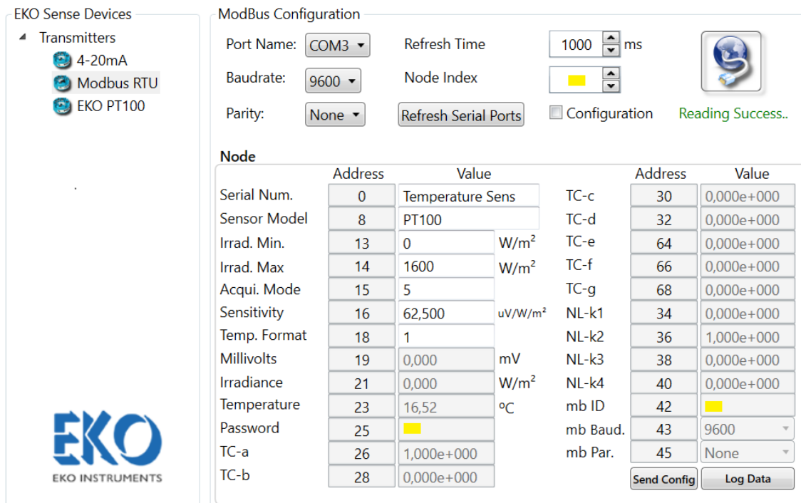
Figura 33. Misura di Temperatura superficiale moduli fotovoltaici su Address 23
