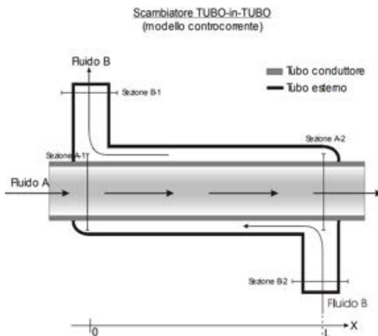
Figura 4-2: Scambiatore di calore tubo in tubo equicorrente (sopra) e controcorrente (sotto) [14]
