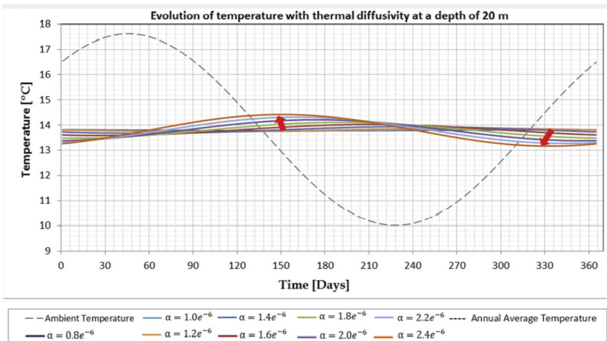
Figura 7-4-C Evoluzione della temperatura del sottosuolo a 20 m per terreni con diversi valori di diffusività termica. il grafico inizia con la stagione estiva [28].
