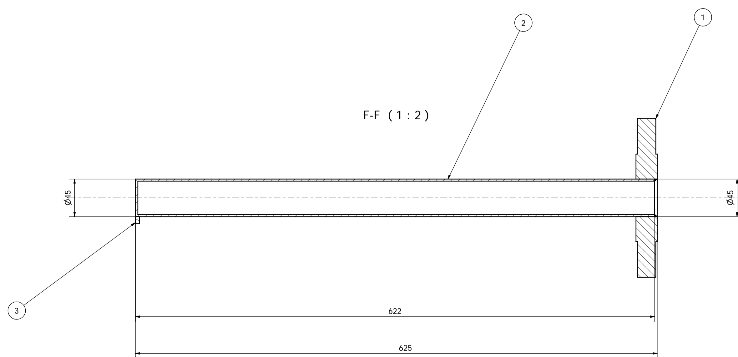
Cartuccia filtrante
