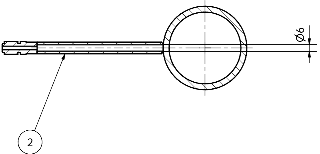
A-A (1:2)
