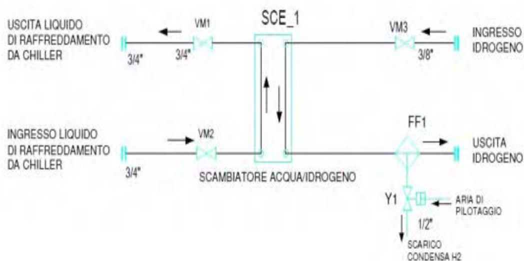
Figura 2.18 - schema del filtro anti umidità per syngas
