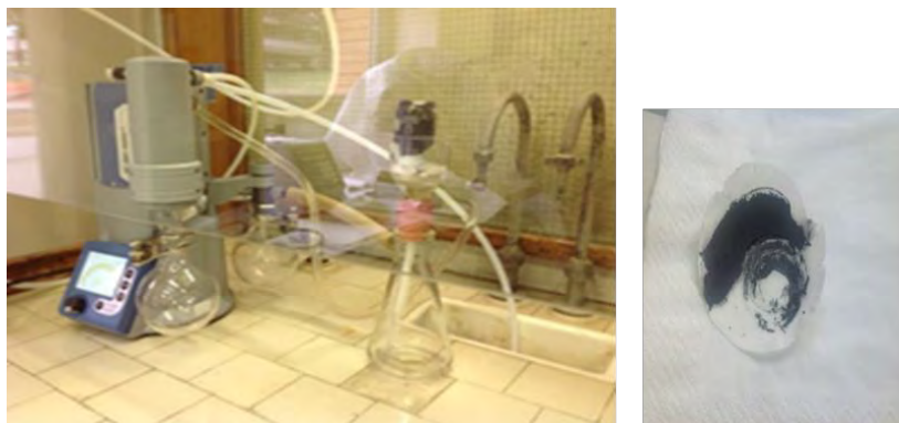
Figura 13. Sistema di filtrazione sotto vuoto e filtro con polvere attiva recuperata
