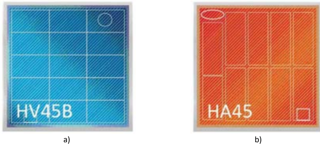
Figura 2.6. Chip LED ad alto voltaggio (HV-LED). a) Chip blu a 15 celle. b) Chip rosso a 10 celle.
