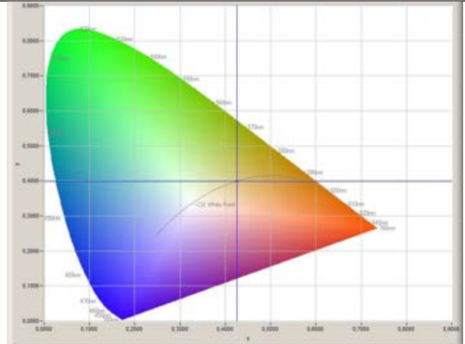
Coordinate cromatiche CIE(x,y)
