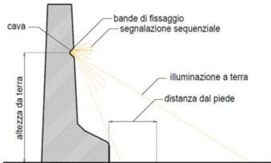
Figura A1.9. Barriera redirettiva a LED
