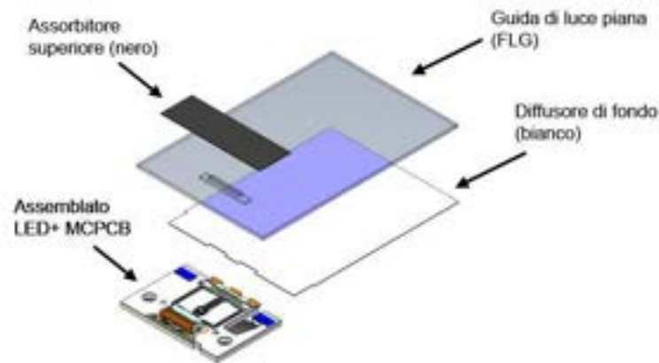
Figura 2.17. LightCell di Oree: superficie SSL sottile e piatta di misura 50x50mm.
