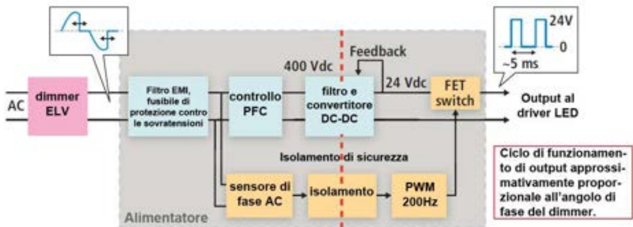
Figura 4.4. Diagramma a blocchi di un alimentatore per il dimming a taglio di fase. Per supportare tale regolazione, un driver LED ha bisogno di componenti aggiuntivi, incluso un sensore di fase AC, un controller PWM e un interruttore MOSFET
