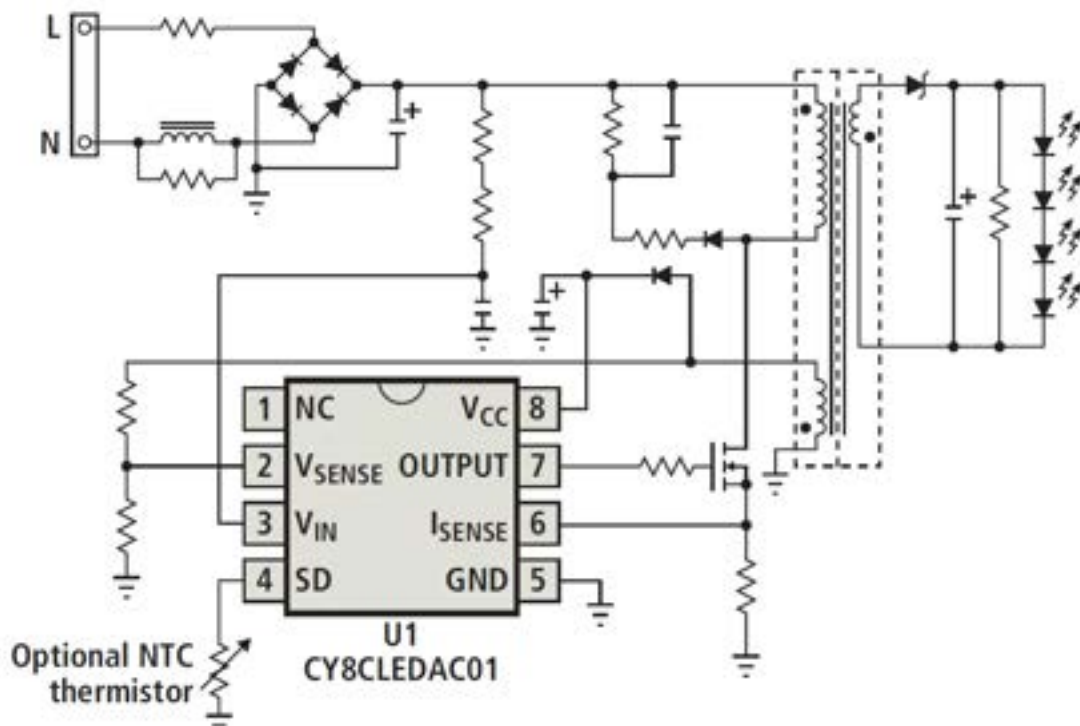
Figura 4.19. Anche in un circuito isolato dove è un trasformatore ad alimentare i LED, il driver può usare il feedback da un winding terziario posto a valle del trasformatore (elemento in grigio) per aggiustare il segnale di alimentazione sulla base delle caratteristiche di funzionamento.
