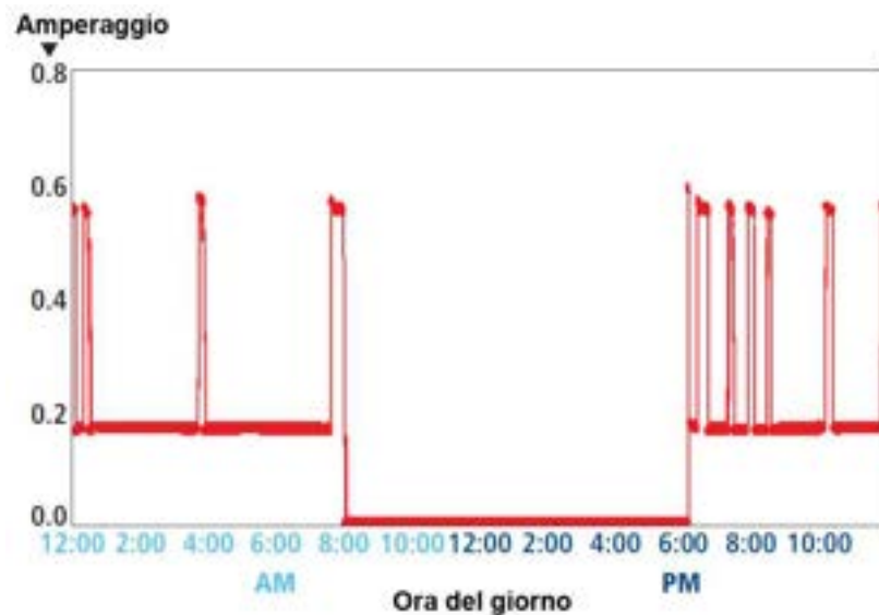
Figura 5.5. Funzionamento di un apparecchio LED nelle 24h nel parcheggio del campus Nike.
