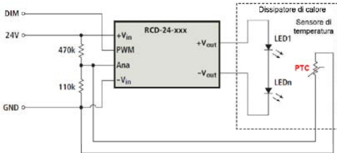
Figura 2.14. Esempio di protezione dal surriscaldamento tramite l'uso di un termistore PTC.
