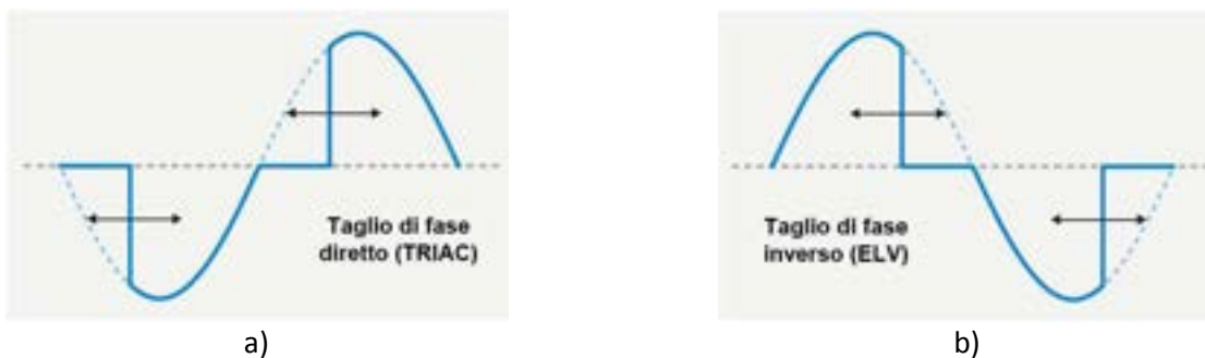
Figura 4.5. I dimmer a taglio di fase riducono la luminosità della lampada tagliando parte della forma d'onda AC. a) Il dimmer TRIAC taglia fuori una porzione della forma d'onda AC nel tratto crescente dell'onda sinusoidale. b) Il dimmer ELV taglia fuori una porzione della forma d'onda AC nel tratto decrescente dell'onda sinusoidale.
