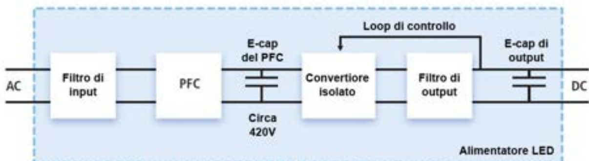
Figura 3.6. I condensatori elettrolitici (E-caps) sono utilizzati quasi in tutti gli alimentatori con input AC, dove svolgono due funzioni principali, cioè all'interno del circuito PFC e nel filtro di output.
