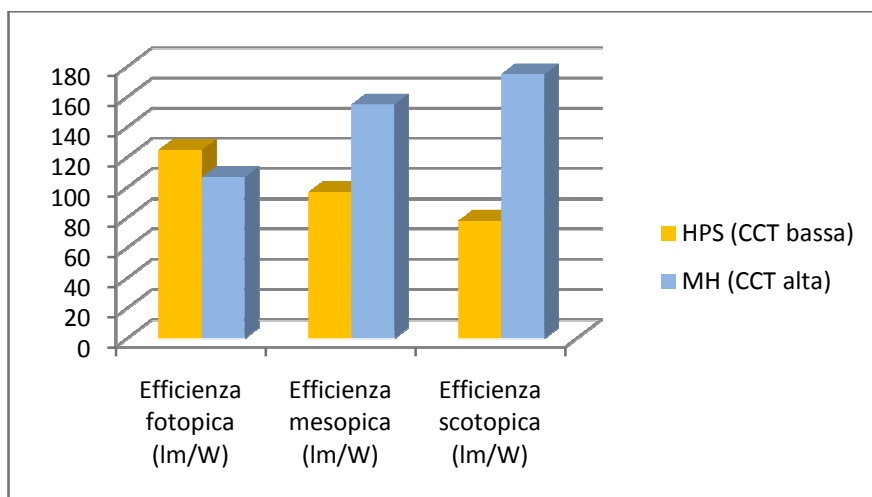
Figura 4.14. Confronto tra le efficienze luminose fotopica, mesopica e scotopica di una sorgente luminosa con CCT elevata (a ioduri metallici, MH) e una con CCT bassa (ai vapori di sodio ad alta pressione, HPS).
