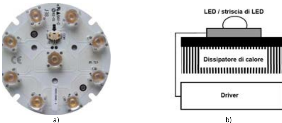
Figura 3.1. a) esempio di engine LED della Future Lighting Solutions. b) schema di un engine LED.
