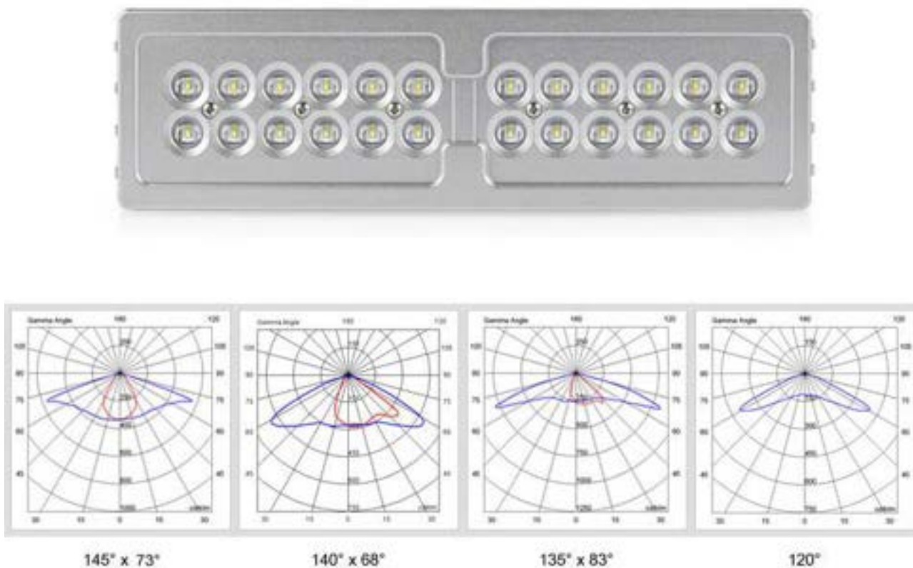
Figura 5.18. Modulo Optoblk della Alliance Optotek Corporation e relative curve fotometriche.
