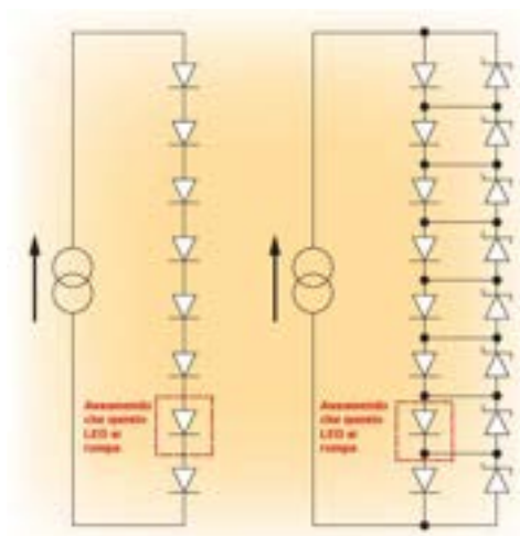
Figura 3.5. In una striscia di LED connessi in serie (sinistra), quando un singolo diodo va in corto circuito, il resto dei LED rimangono accesi e la corrente rimane stabile. Tuttavia, se un LED va in circuito aperto, tutti i LED si spengono, a meno che la striscia non sia protetta da componenti aggiuntivi. Tale protezione, ottenuta ad esempio utilizzando un diodo zener in parallelo con ogni LED (destra), aggiunge costo e complessità.
