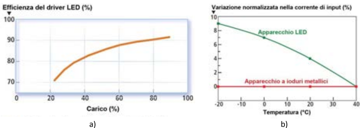
Figura 5.1. Corrente di input fornita da un driver LED.
