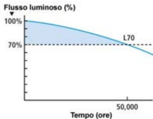
Figura 4.15. Molti apparecchi LED sprecano energia (area evidenziata in azzurro) perché inizialmente hanno un flusso superiore a quello richiesto per bilanciare il decadimento del flusso ed assicurare una L70 sufficientemente lunga.
