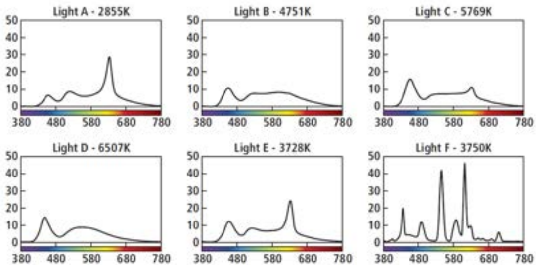
Figura 6.17. Gli spettri delle sei condizioni luminose testate.
