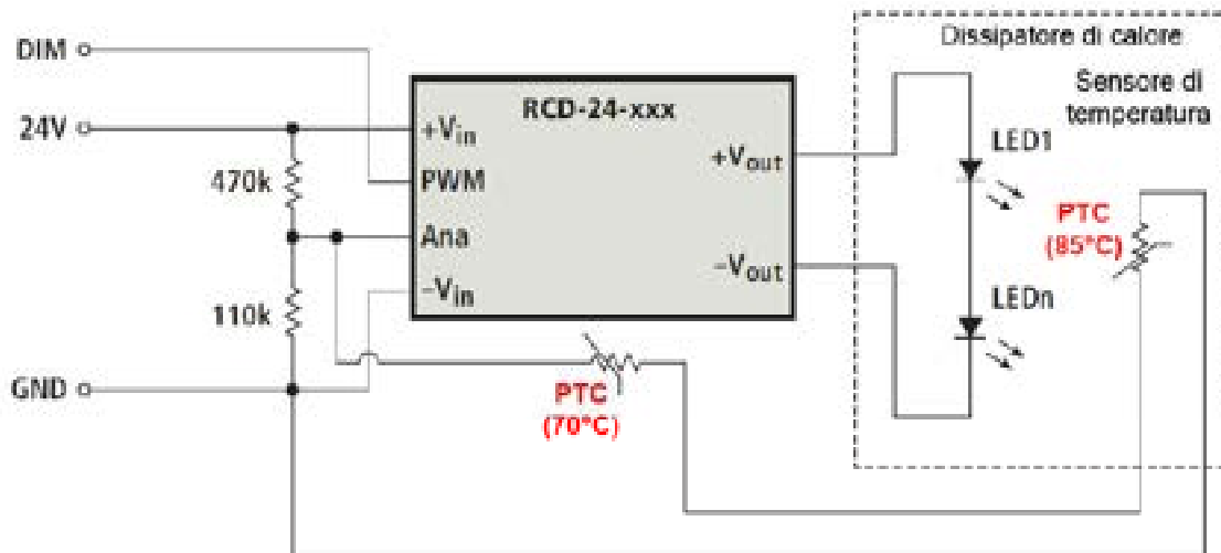
Figura 2.15. Utilizzando due termistori PTC si possono proteggere dal surriscaldamento sia il LED che il driver.
