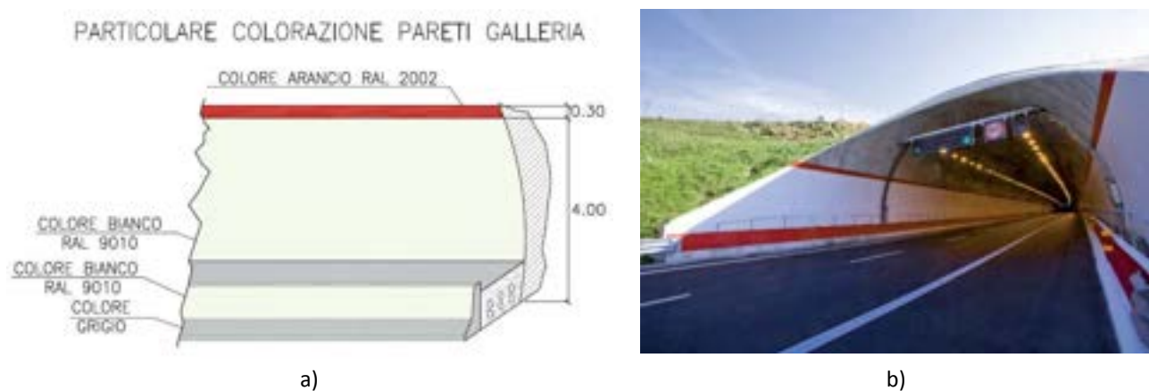
Figura A1.6. Colorazione della superficie interna di una galleria tipo.
