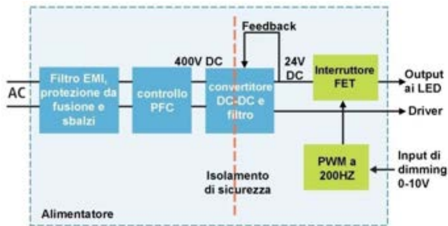
Figura 4.3. Il dimming PWM è inoltre applicabile a scenari di controllo di tipo 0-10V, ma richiede un controller PWM che comandi l'interruttore di output MOSFET di un alimentatore che in risposta alimenta in corrente continua un driver LED.
