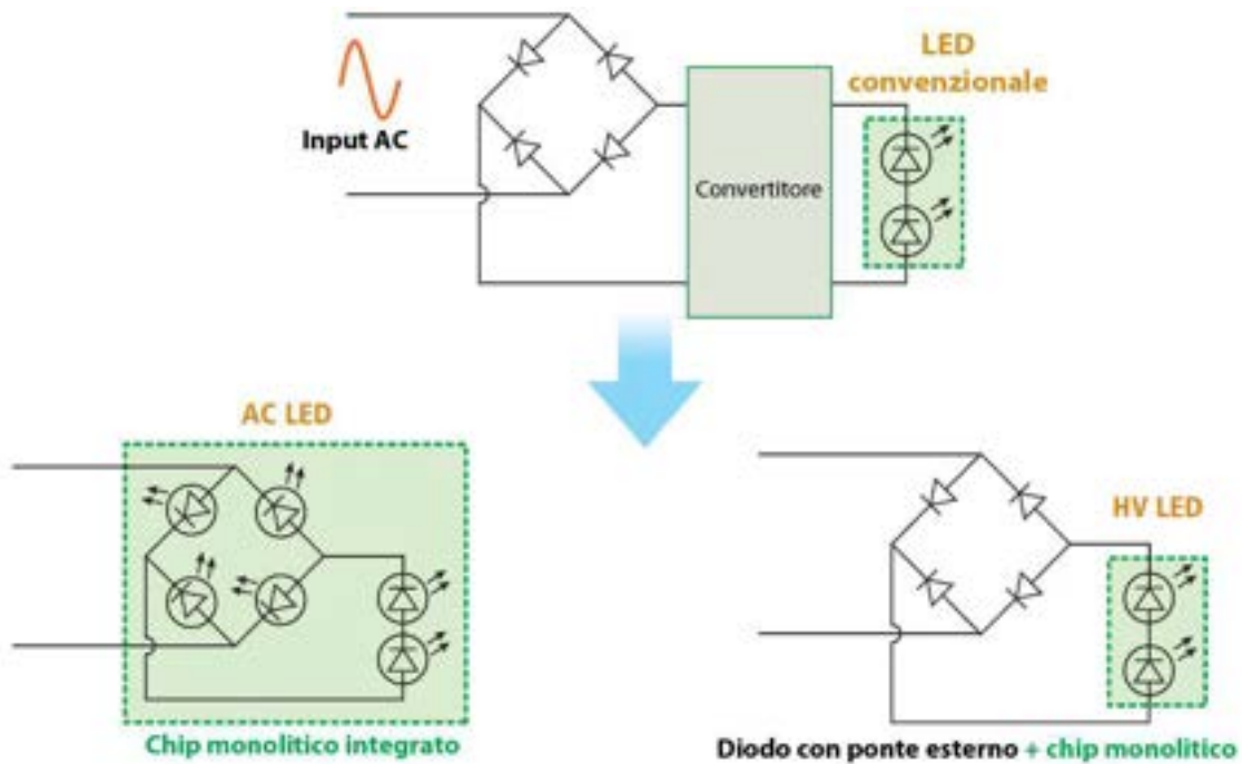
Figura 2.7. Confronto tra un LED convenzionale, un LED AC e un LED HV. Il LED AC presenta un rettificatore integrato dell'alimentazione AC, ma l'utilizzo del LED è solo il 50-70% poiché tutte le celle LED non emettono luce continuamente quando il LED è acceso. Il LED HV richiede un rettificatore esterno a ponte, ma tutte le celle LED sono sempre accese. Né il LED AC né quello HV richiedono un driver LED.
