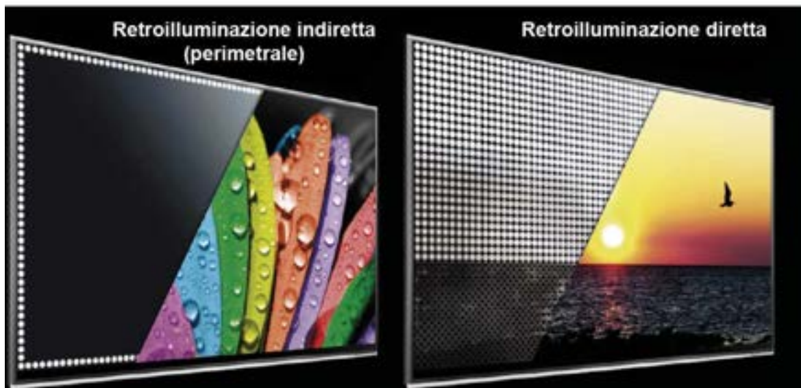
Figura 6.7. Le due principali tecniche di retroilluminazione LED: retroilluminazione indiretta, con diodi posizionati sui bordi dello schermo e guida di luce che distribuisce il flusso e retroilluminazione diretta, con diodi posizionati dietro lo schermo.
