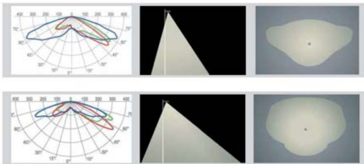
Figura A1.14. Apparecchio Edge Tunnel di Ruud Lighting impiegato per la Galleria Veilino e per la galleria Pregasina.
