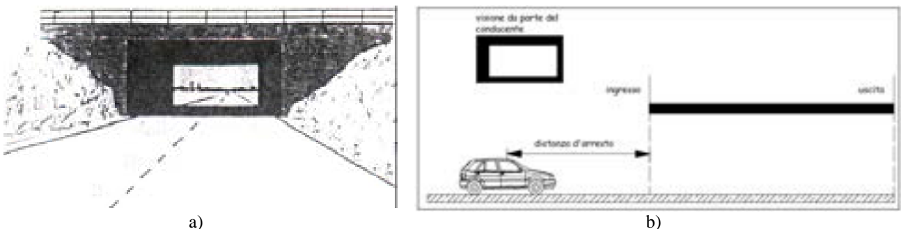
Figura A1.5. Galleria corta visione d'ingresso (a) e sezione (b).
