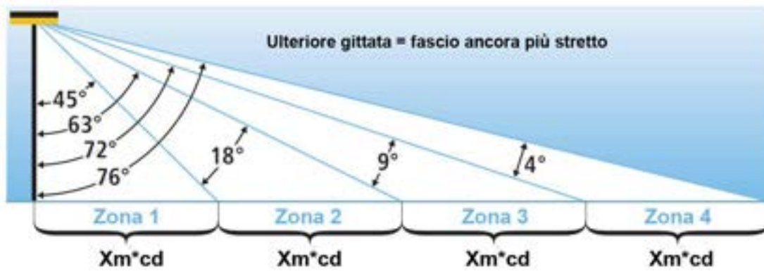
Figura 5.8. Gli apparecchi per illuminazione stradale devono emettere più luce con fasci sempre più stretti per illuminare uniformemente aree che sono progressivamente più lontane da esso. Ciò genera problemi di abbagliamento.
