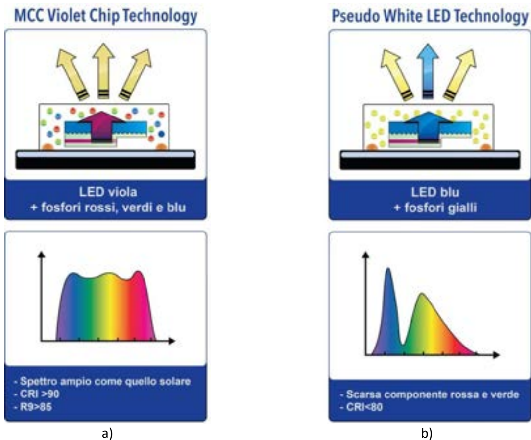
Figura 2.16. La Mitsubishi Chemical Corporation ha prodotto i LED “Natural Vision Lighting”, con chip viola e fosfori RGB. La distribuzione spettrale molto diversa dai comuni LED bianchi consente una resa cromatica molto alta e l’assenza di binning, perché il colore della luce dipende dai fosfori e non dal LED.
