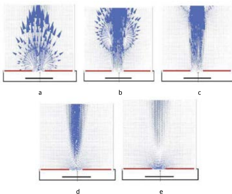
Figura 2.11. Vettori di velocità del flusso a getto artificiale non appena viene espulsa l'aria.
