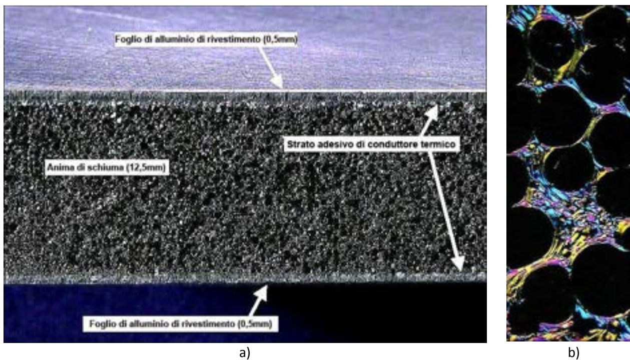
Figura 2.9. Schiuma di grafite per dissipatori di calore sviluppata dall'ORNL.
