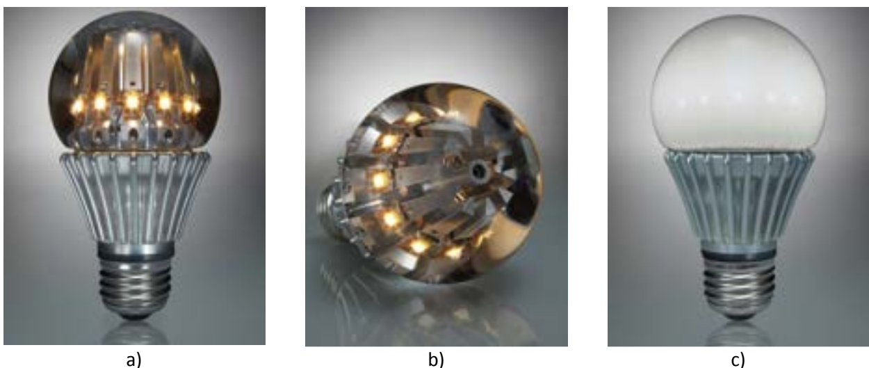
Figura 2.10. a) e b) Prototipo del bulbo LED per retrofitting da 75W presentato da Switch Lighting. c) Bulbo LED così come verrà commercializzato, con un globo in vetro smerigliato diffondente.
