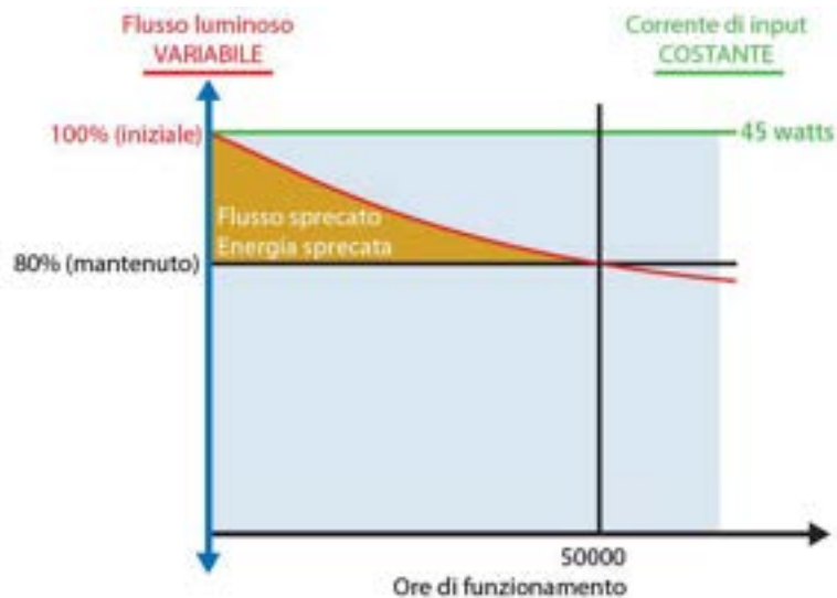
Figura 4.16. Grazie ai sistemi di illuminazione intelligente è possibile adattare l'alimentazione (curva rossa) per fornire un flusso luminoso costante (linea orizzontale nera) evitando sprechi energetici.
