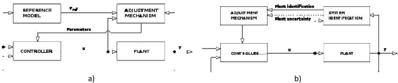
Figura 4.9. Sistemi di controllo adattivo a confronto. a) MRAC (Model Reference Adaptive Control). b) MIAC (Matrix Industrial Automotive Controller).
