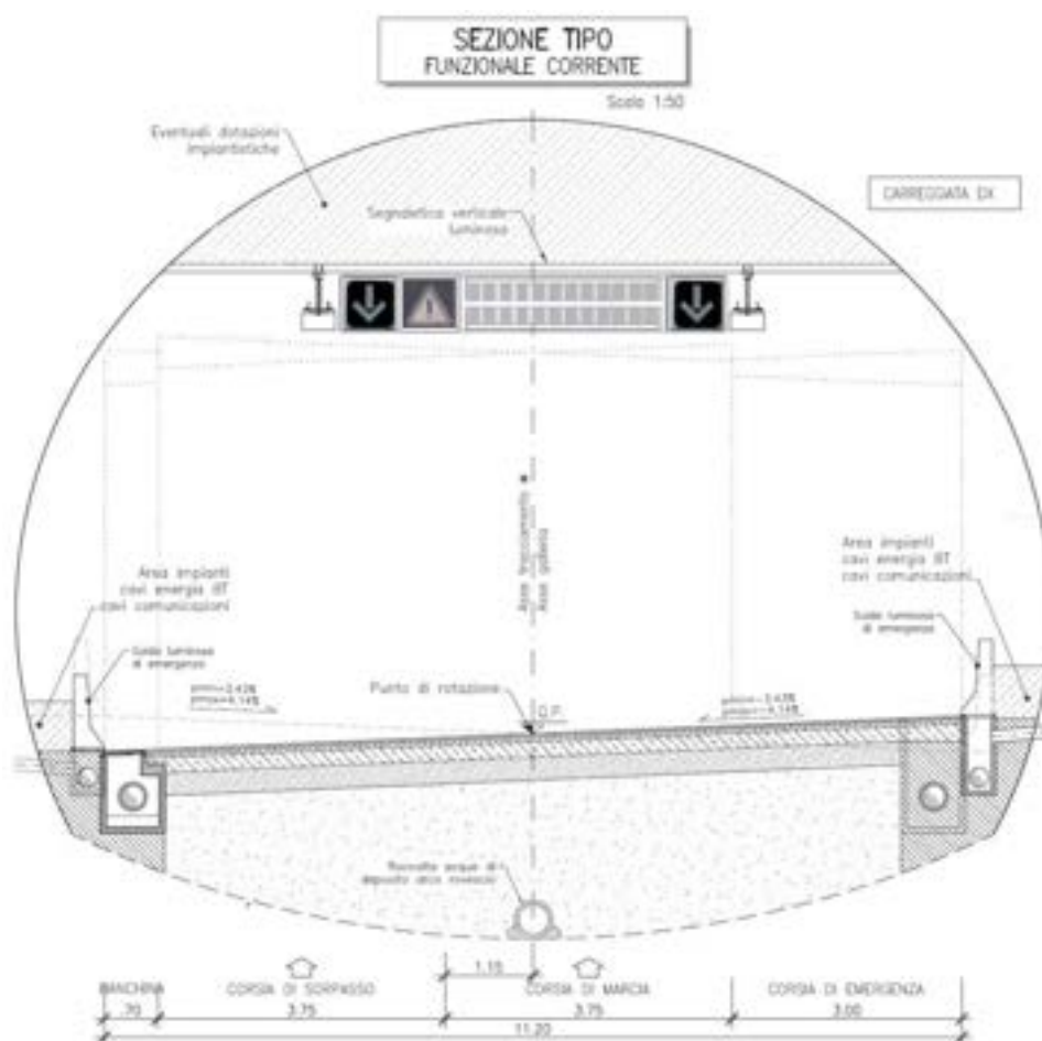
Figura I.8. Sezione tipo di una galleria stradale
