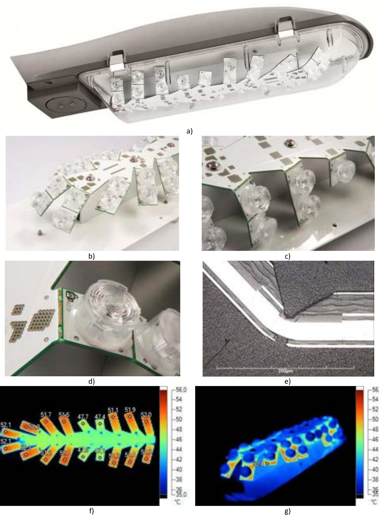
Figura 5.24. Shröder Lighting ha integrato la tecnologia HSMtec printed-board di Hausermann GmbH nello sviluppo di un nuovo apparecchio stradale.
