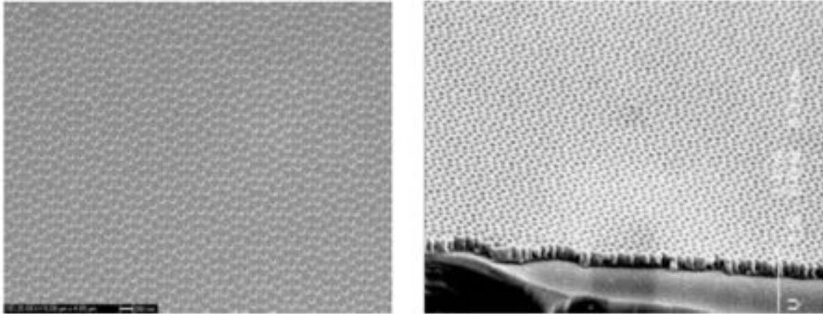
Figura 2.5. Misure SME di una texturizzazione quasi-cristallina stampata su un epistrato di GaN. La texturizzazione copre l'intera superficie malgrado i difetti di crescita mostrati a destra. Il diametro del foro è di 90nm.
