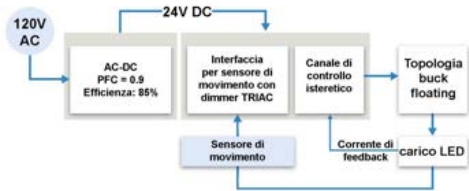
Figura 4.20. Modello a blocchi di un prototipo di lampada LED per retrofitting che dimostra come caratteristiche come i sensori di movimento possano aggiungere valore all'apparecchio.
