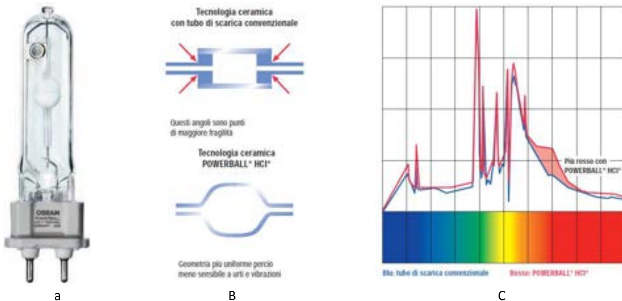
Figura 1.5. Lampada a ioduri metallici in tecnologia ceramica.
