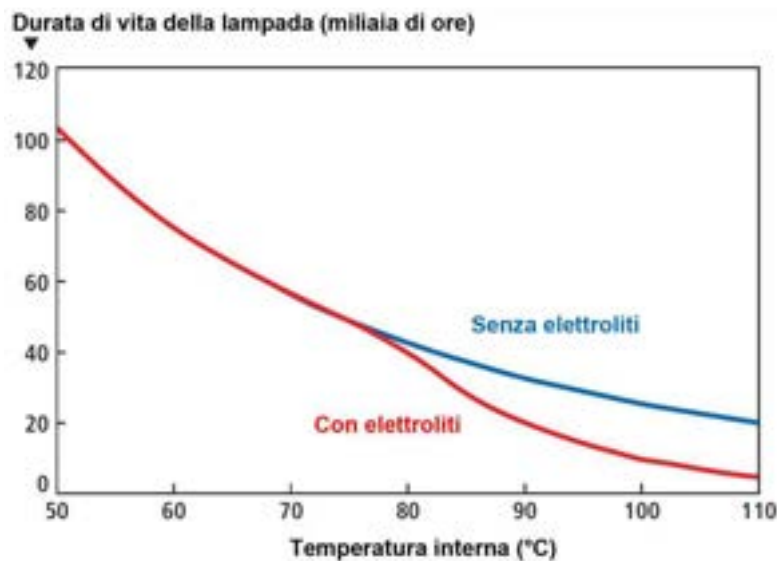
Figura 6.3. Durata di vita di una lampada LED al variare della temperatura in presenza e in assenza di capacitori elettrolitici.
