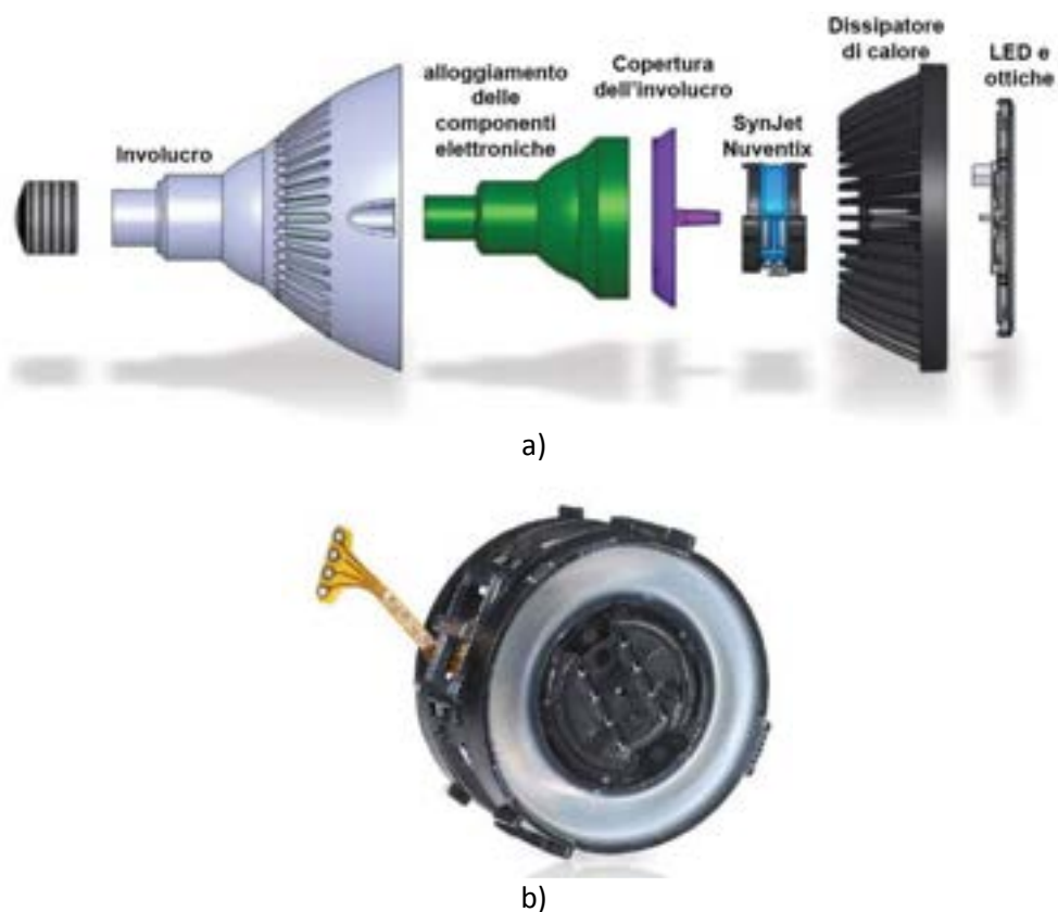
Figura 2.12. Raffreddamento attivo.
