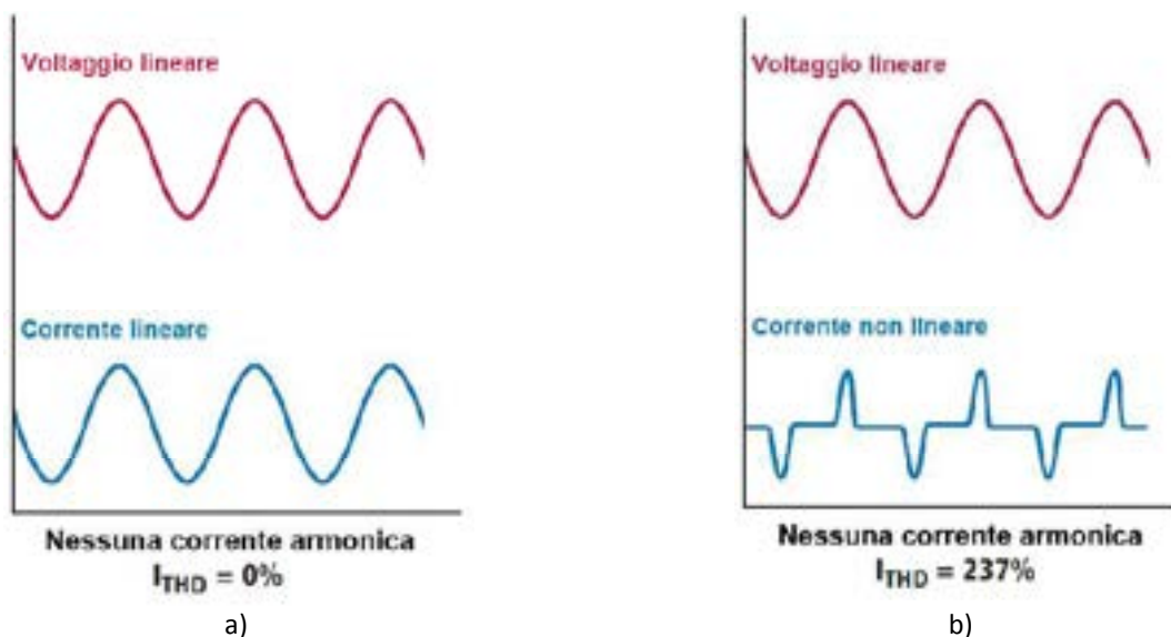
Figura 4.6. Carichi elettrici lineari e non lineari.
