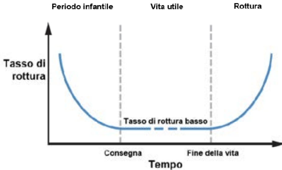
Figura 3.3. Curva che rappresenta il tasso di rottura dei LED nel tempo.
