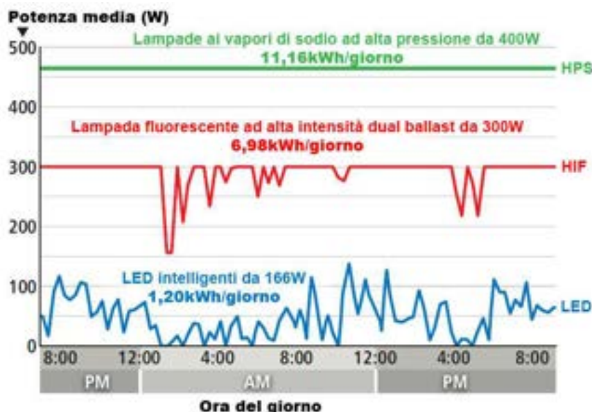
Figura 4.10. Consumo medio di un apparecchio tradizionale ai vapori di sodio ad alta pressione, di un apparecchio fluorescente ad alta intensità di tipo dual ballast e di un apparecchio LED all'interno di un sistema di illuminazione intelligente.
