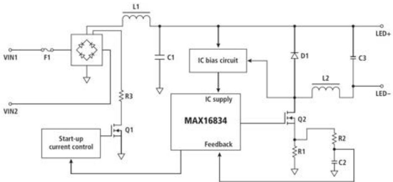
Figura 6.6. Diagramma a blocchi di un driver LED privo senza capacitore elettrolitico.
