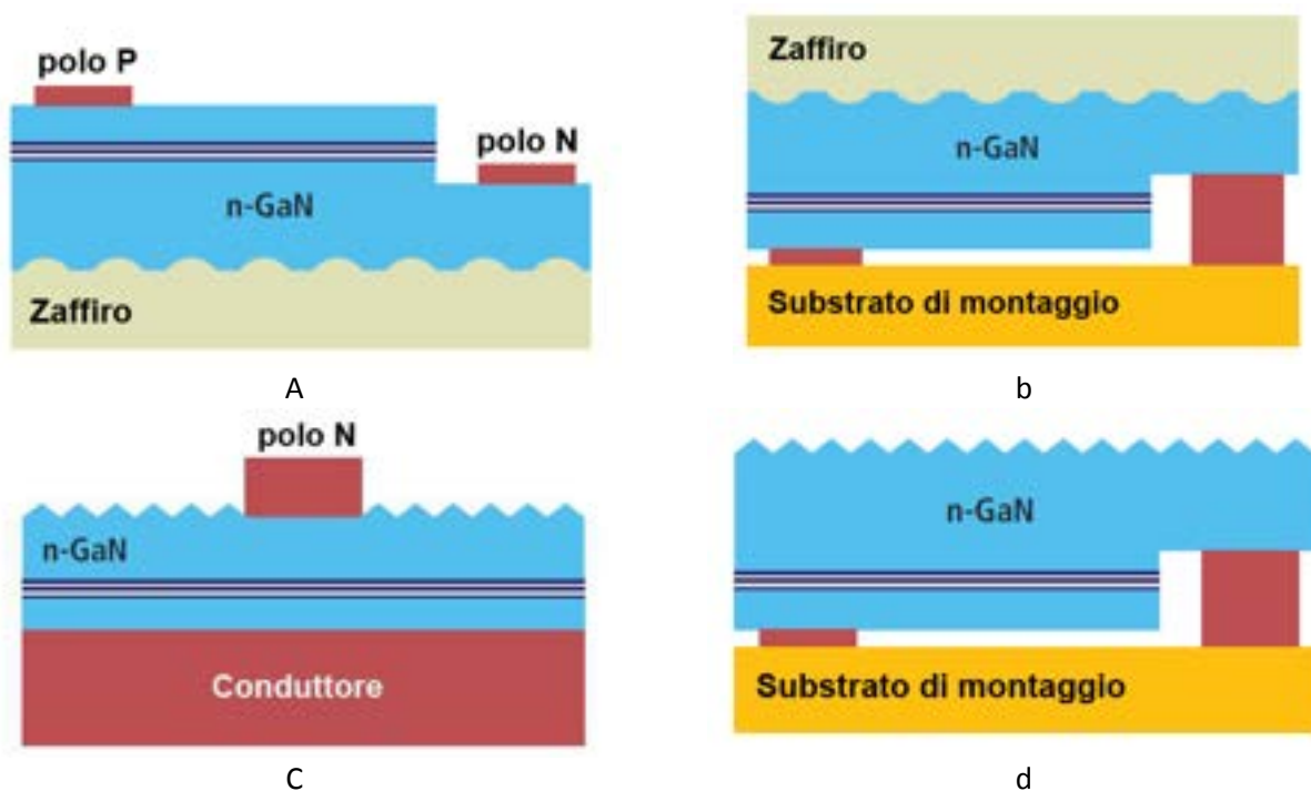
Figura 2.4. Strutture dei chip LED che utilizzano la nano-texturizzazione delle superfici.
