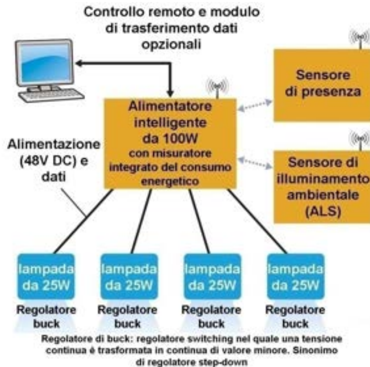
Figura 4.17. In questo sistema di illuminazione intelligente relativamente costoso, ogni apparecchio illuminante include un alimentatore AC/DC e una ricetrasmittente per il collegamento wireless al network di controllo.
