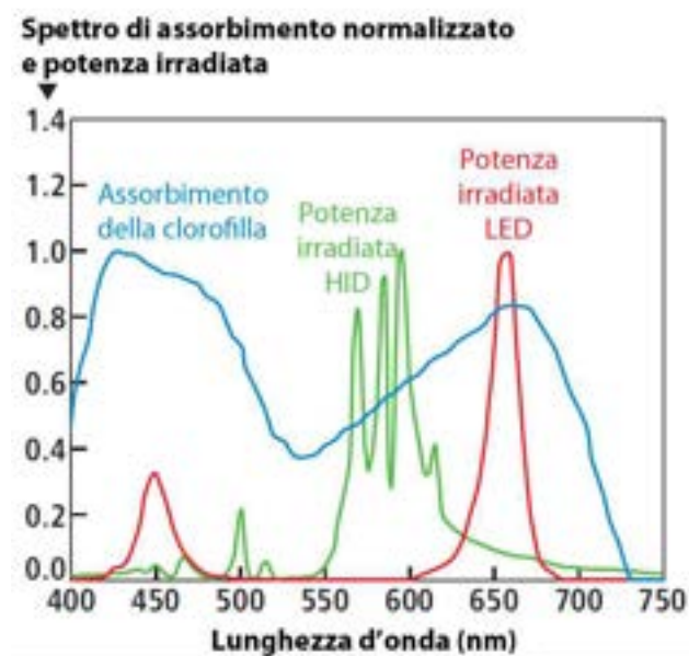
Figura 6.9. I LED possono essere scelti per corrispondere esattamente alla curva di assorbimento della clorofilla.
