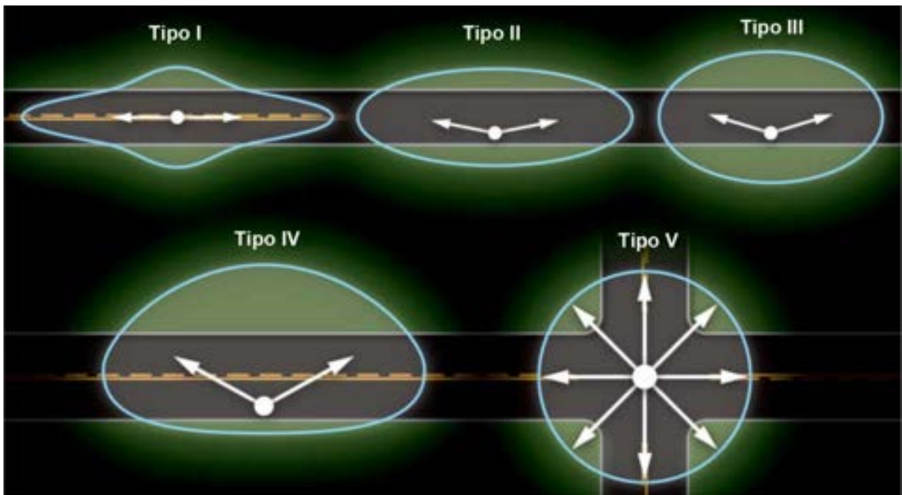
Figura 5.7. Tipi di distribuzione luminosa per apparecchi stradali secondo la classificazione effettuata dalla IESNA (Illuminating Engineering Society of North America)
