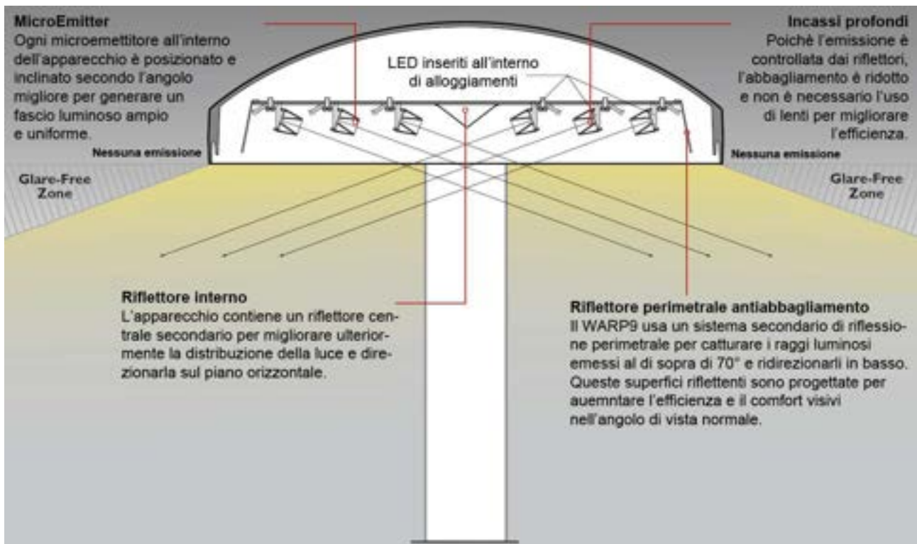
Figura 5.26. Sezione schematica illustrante il funzionamento dell'apparecchio Warp9 della Kim.
