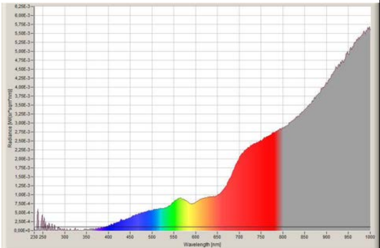
Spettro di emissione
