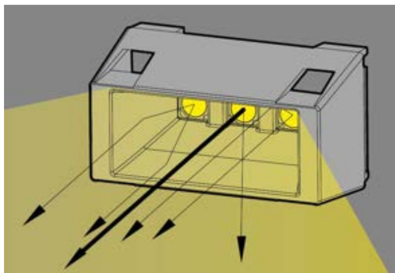
Figura 5.27. Schema del MicroEmitter.
