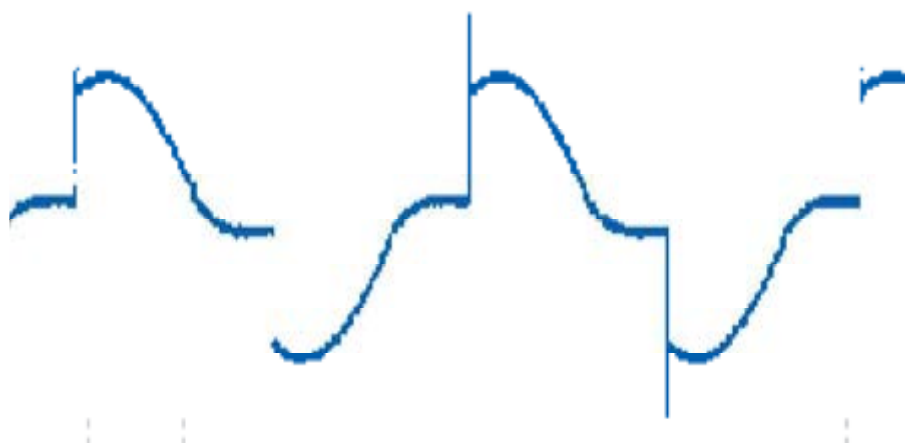
Figura 6.4. Voltaggio di output tipico (asse verticale) nel tempo (asse orizzontale) per un dimmer TRIAC.
