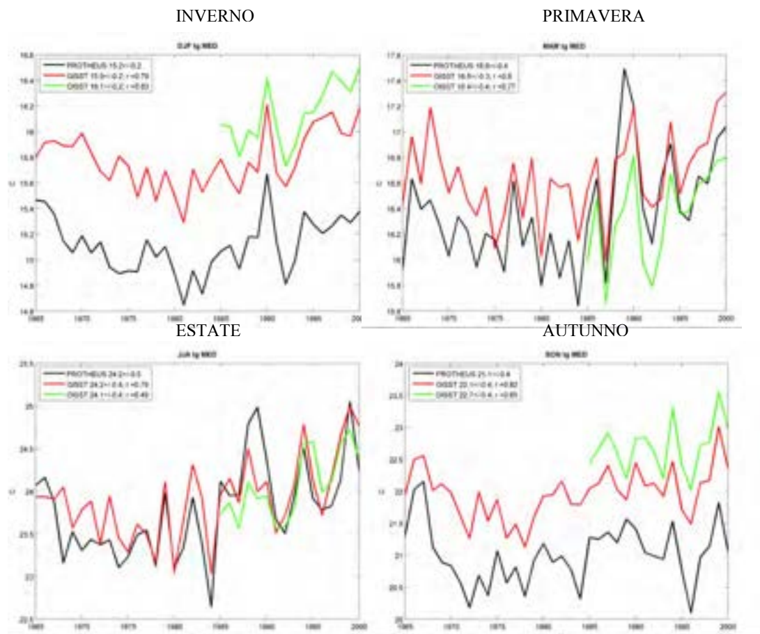
Figura 2: TSM stagionale del bacino Mediterraneo ( ^{\circ}\text{C} ) in CPL (PROTHEUS, linea nera) e negli archivi osservati GISST 2.3 (linea rossa) and OISST (linea verde). L'archivio GISST 2.3 è anche usato come condizione al bordo superficiale per la simulazione atmosferica RCM. La legenda della figura riporta anche il valore medio con la corrispondente deviazione standard per il periodo comune 1985-2000, e il coefficiente di correlazione r tra le osservazioni e la simulazione accoppiata CPL.
