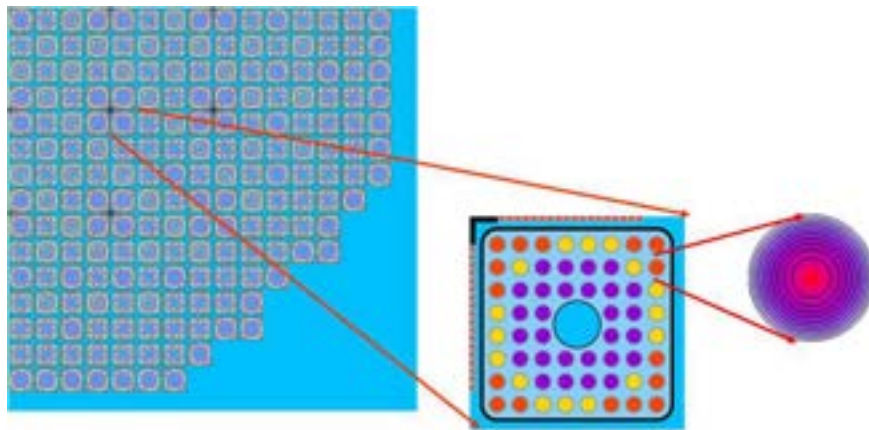
Fig. 5-14 Simulazione SIMULATE-3K
