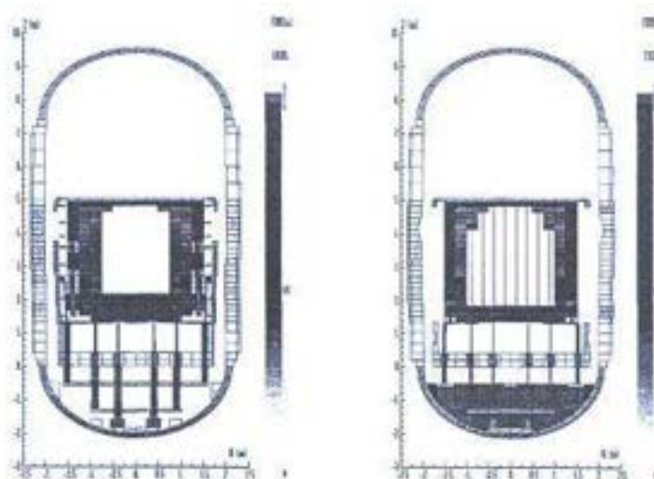
Fig. 5-25 Distribuzione materiale e liquido a 19000 e 23000 sec. del transitorio di un PWR 900 MWe con il codice ICARE2
