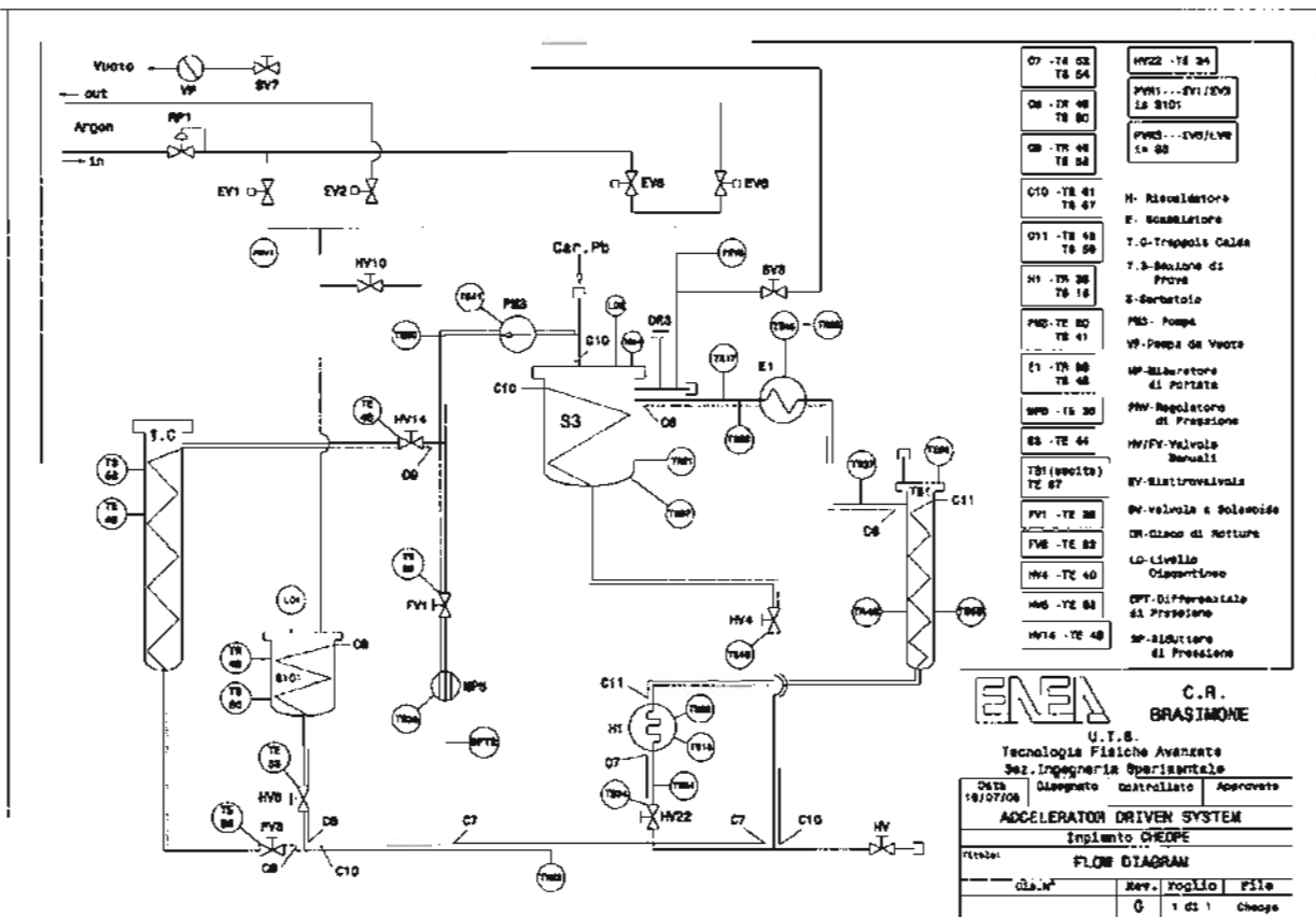
Fig. 2 P&I della facility CHIEOPE III [7].
