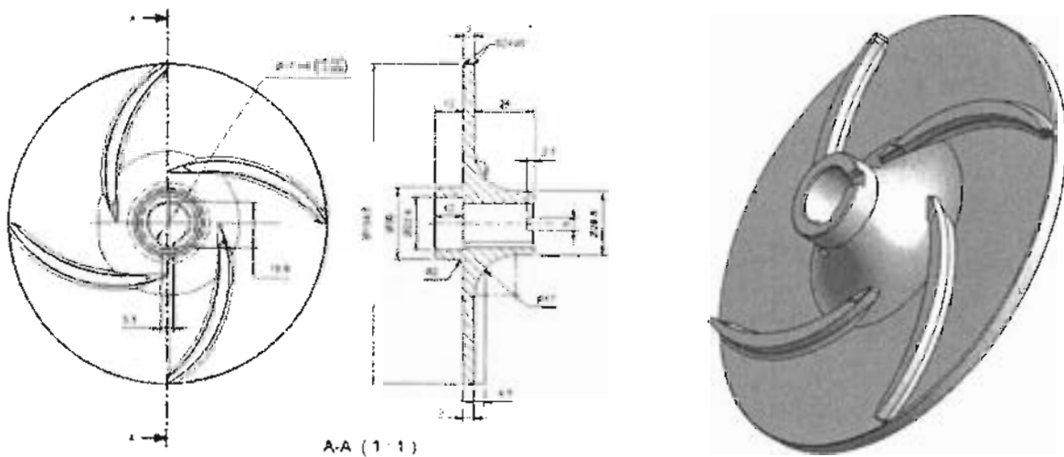
Fig. 11 Disegno mediante CAD della girante VII40.
