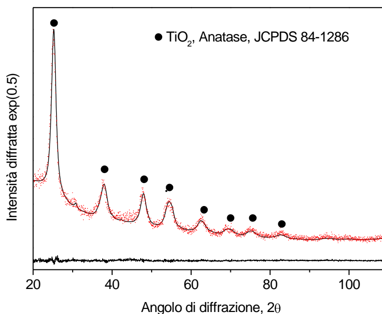
Figura 9: Analisi XRD e profilo calcolato mediante il metodo di Rietveld relativi al campione \text{TiO}_2 1 M in TTIP (temperatura di idrolisi 25^\circ\text{C} , temperatura di calcinazione 200^\circ\text{C} ).
